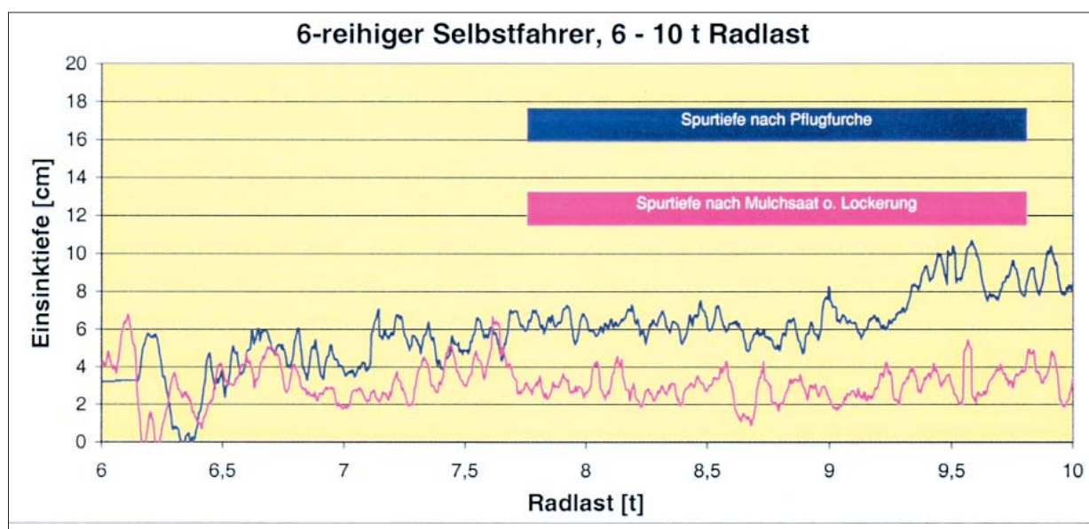
Abb. 19: Spurtiefe eines Rübenroders bei zunehmender Bunkerfüllung und nach unterschiedlicher Bodenbearbeitung
