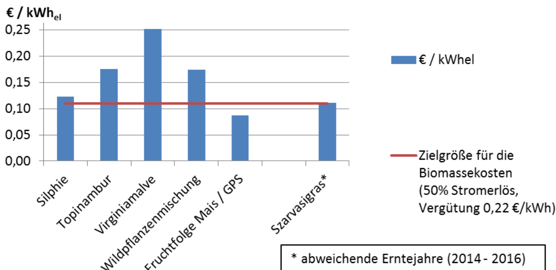
Abbildung 3: Biomassekosten (€/kWh el ) der geprüften Kulturen im Mittel der 5 Standorte
